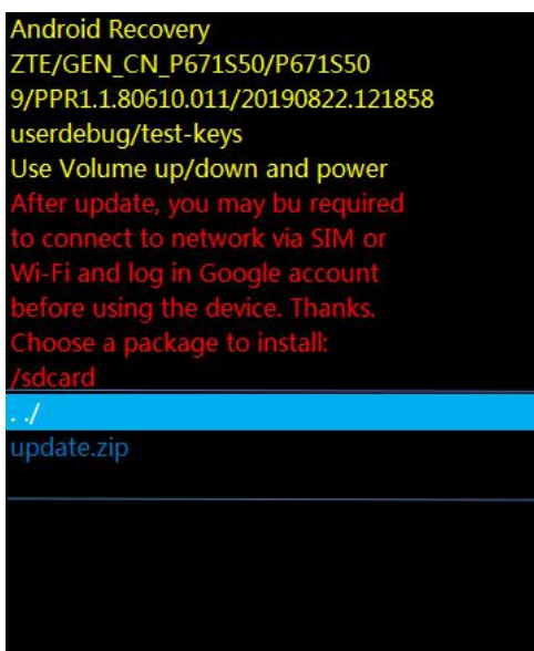
图 3-3 SD 卡目录
